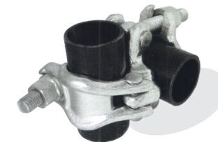
DOUBLE COUPLER USA TYPE FOR TUBE OD 48.3mm (EN-74 / BS 1139)
